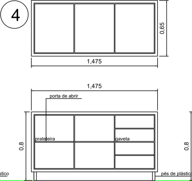
4 Balcão Cozinha Profundidade 50cm
