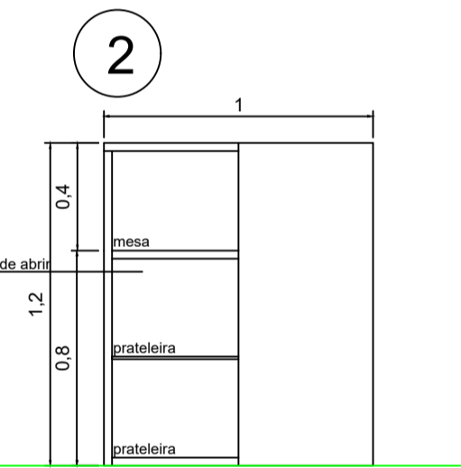
2 balcão recepção 1 profundidade 50cm
