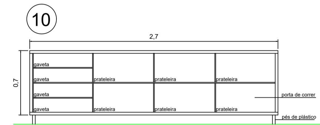
10 sala de curativo profundidade 58.9cm
