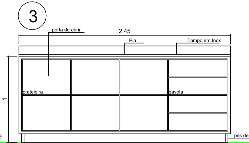
3 balcão Sala de Lavagem profundidade 50cm
