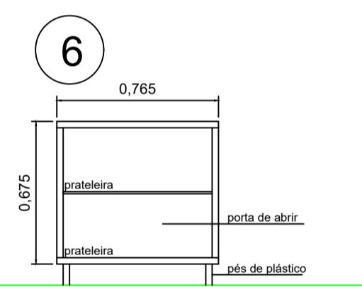
6 banheiro funcionários 2 profundidade 53cm
