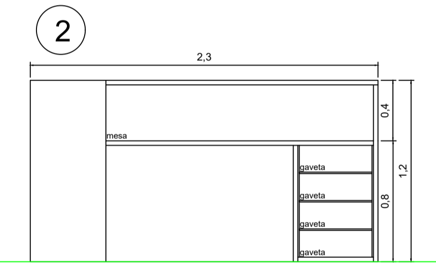
2 balcão recepção 2 profundidade 50cm
