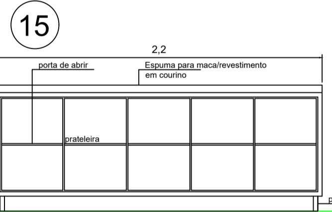
15 Maca Sala de Vacina Profundidade 50cm
