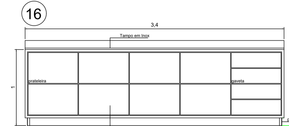
16 balcão Sala de Esterelização profundidade 50cm
